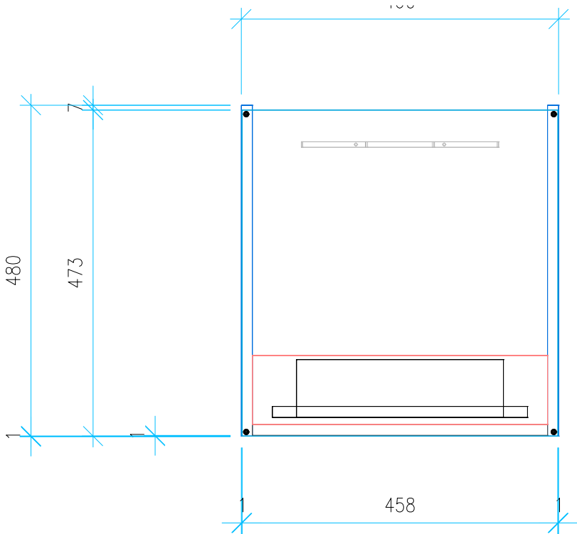
Ansicht 4 / Vorderansicht
