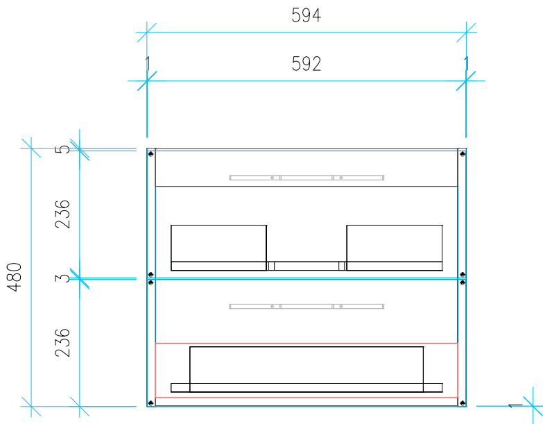
Ansicht 4 / Vorderansicht
