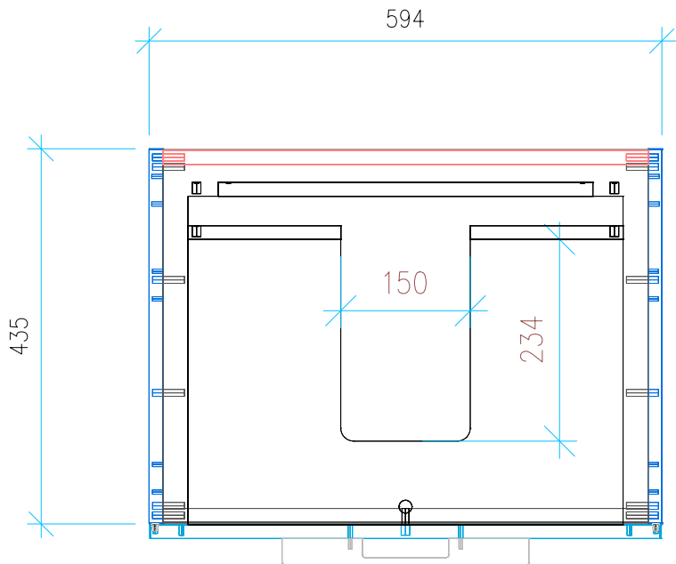
Ansicht 2 / Draufsicht
