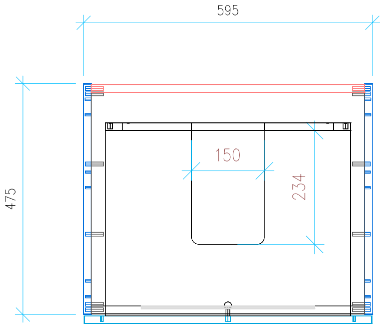
Ansicht 2 / Draufsicht
