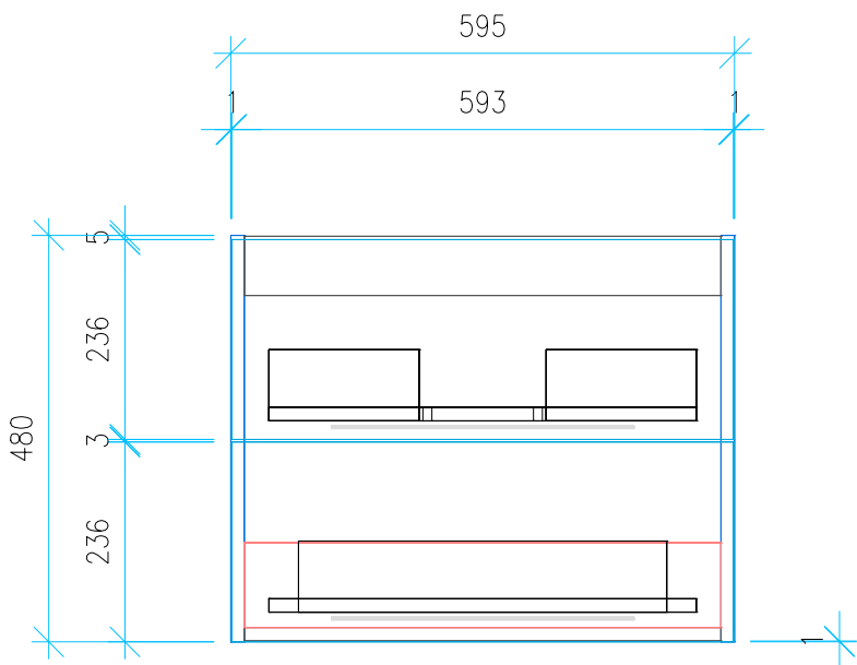
Ansicht 4 / Vorderansicht
