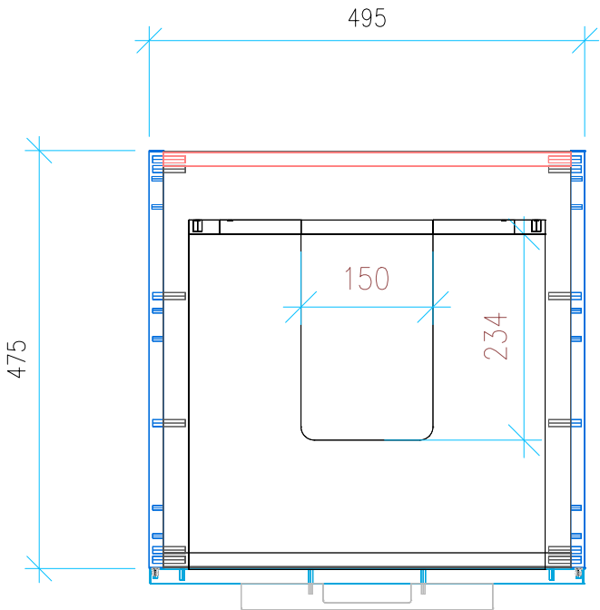
Ansicht 2 / Draufsicht
