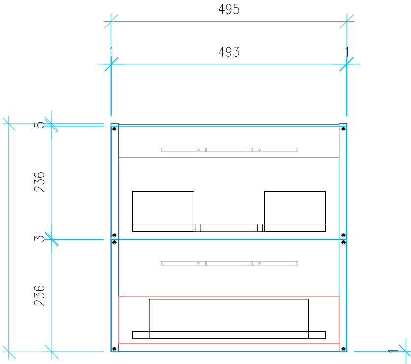
Ansicht 4 / Vorderansicht
