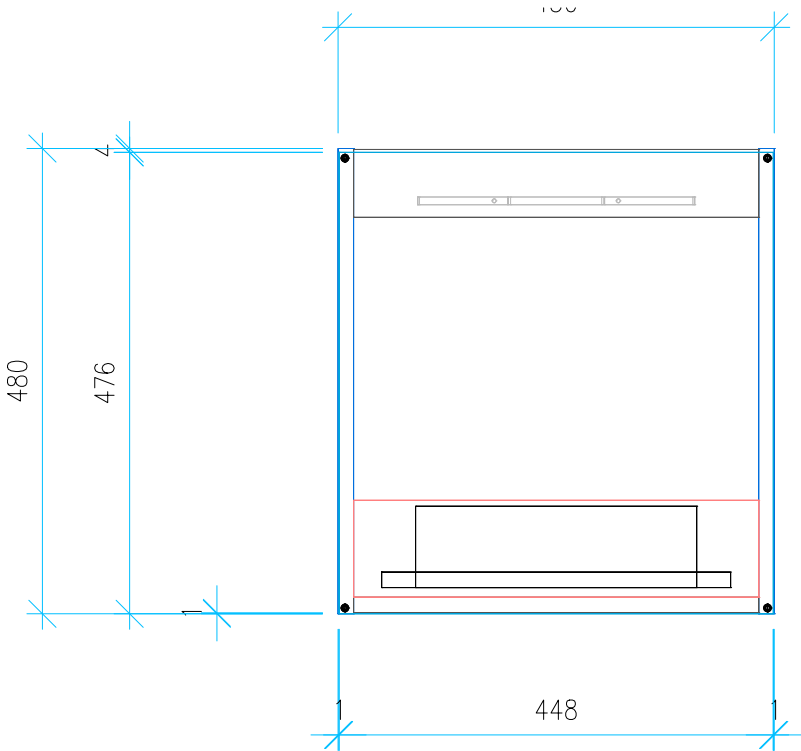
Ansicht 4 / Vorderansicht
