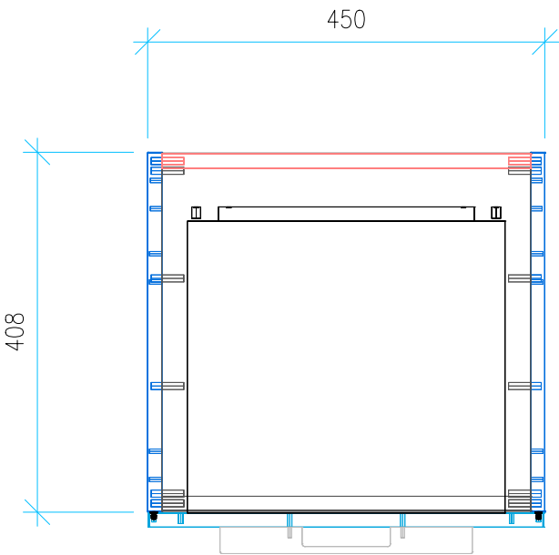
Ansicht 2 / Draufsicht
