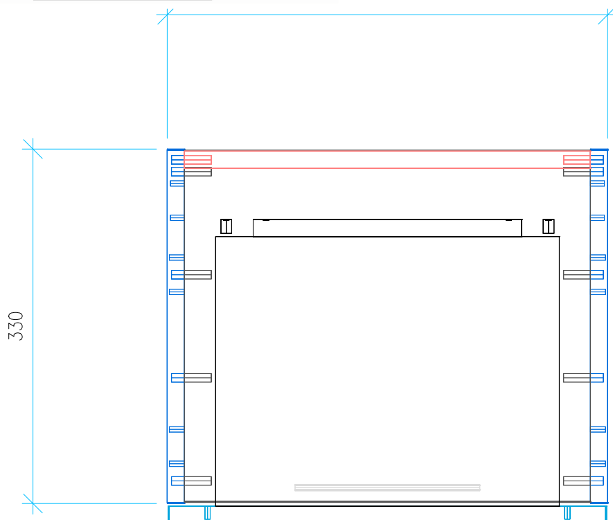
Ansicht 2 / Draufsicht
