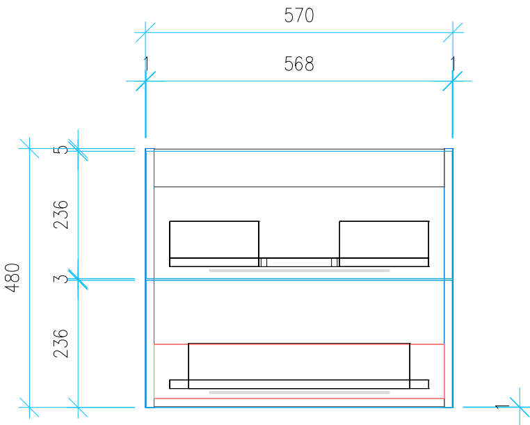
Ansicht 4 / Vorderansicht
