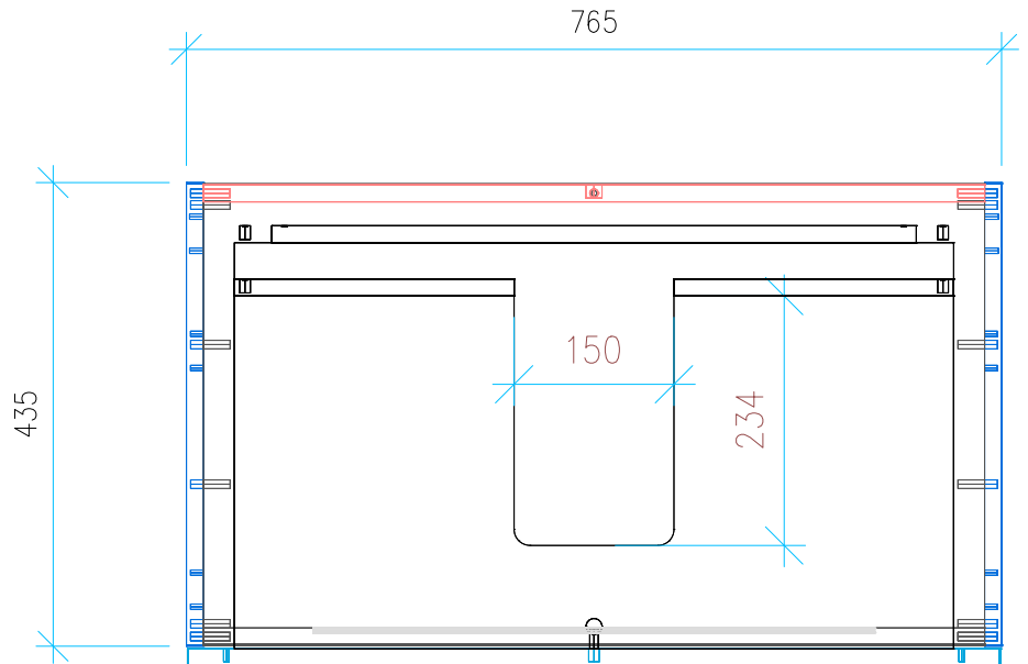
Ansicht 2 / Draufsicht
