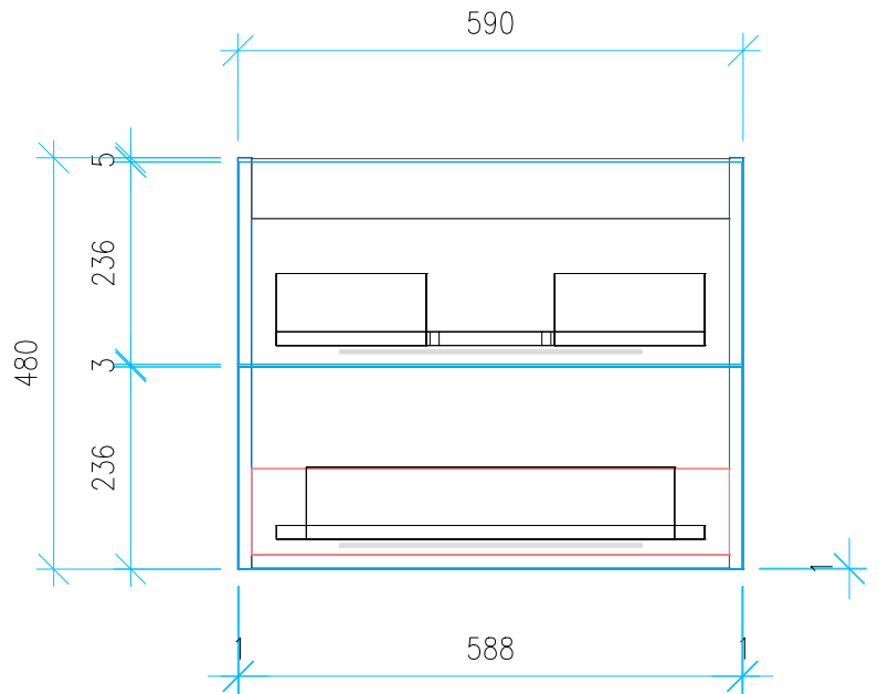
Ansicht 4 / Vorderansicht
